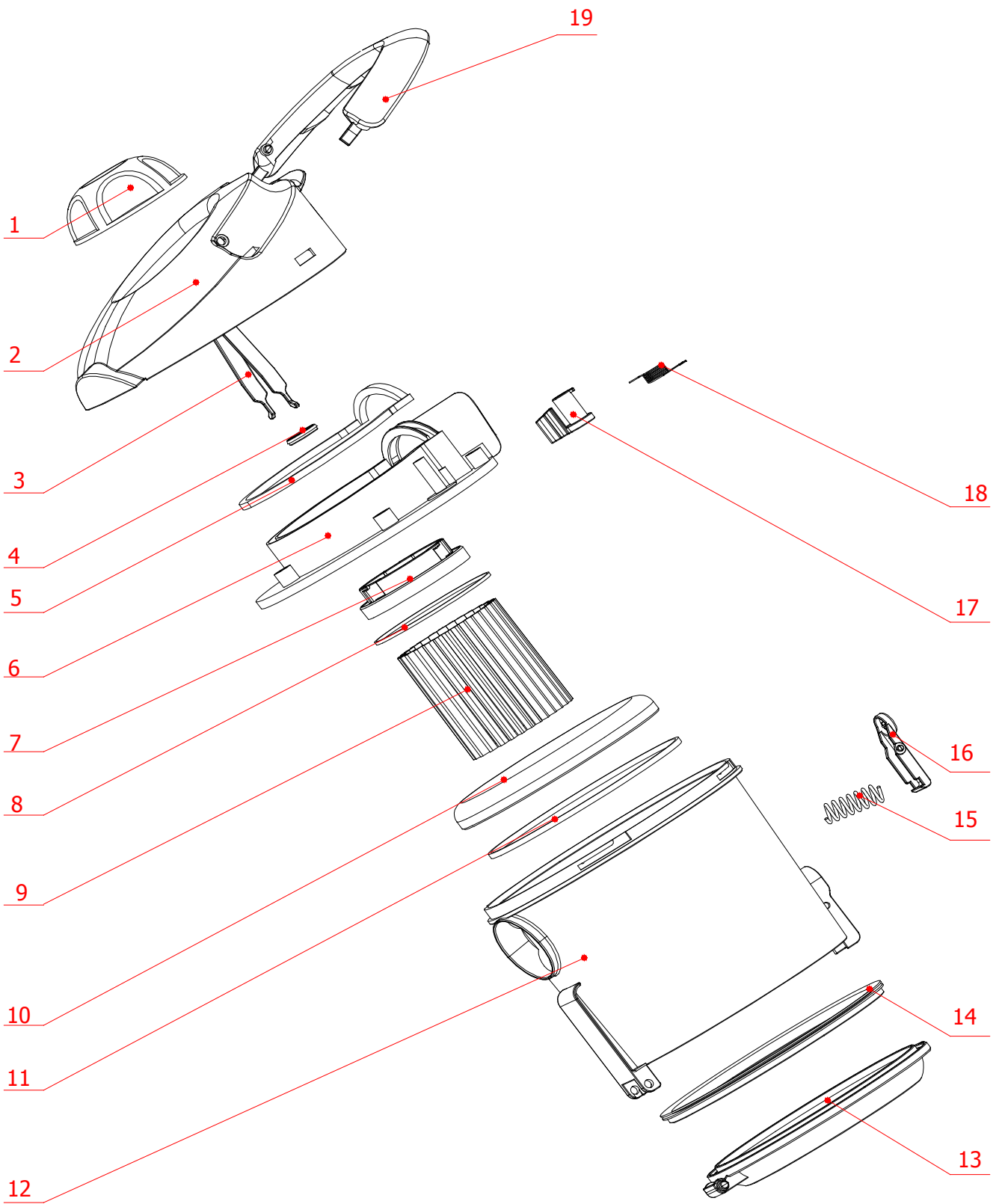
EXPLODER FOR VC-T4002E
